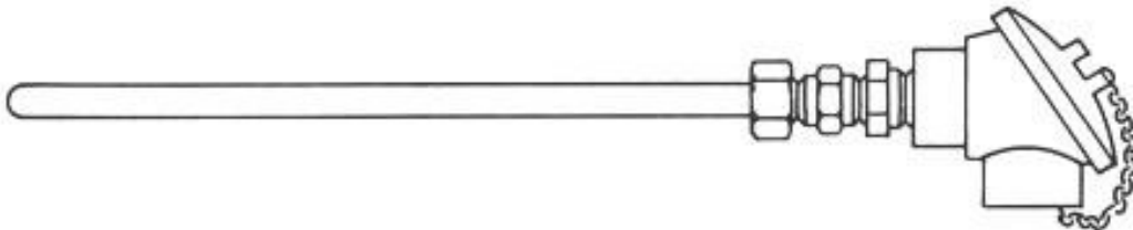
TERMOPAR O RTD CON FUNDA PROTECTORA (TUBING AC. INOX) CON CABEZA DE CONEXIONES (A4)
